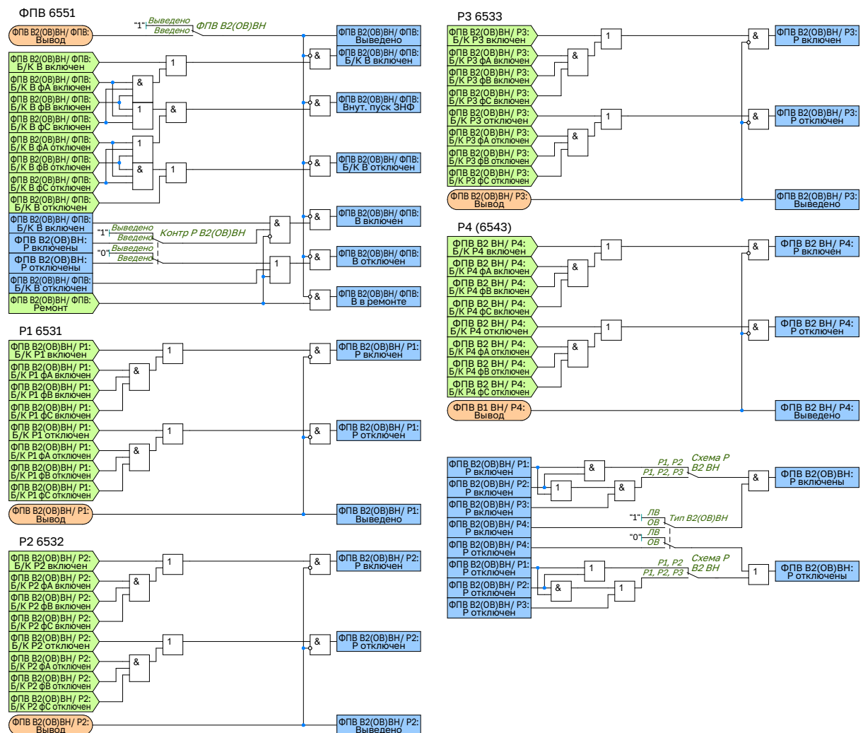
Рисунок 2.45 – Функциональная схема логики ФПВ В2(ОВ) ВН
