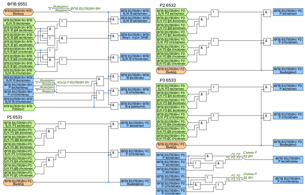
Рисунок 2.44 – Функциональная схема логики ФПВ В1(ЛВ) ВН
